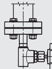
12 Conexión bridada con válvula de descarga
