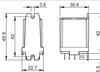
056.26 con relé
