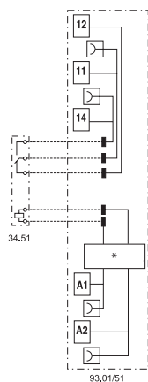
* Circuito de protección y señalización
