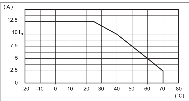
F L78-11 Corriente de salida en función de la temperatura ambiente (78.2E)
