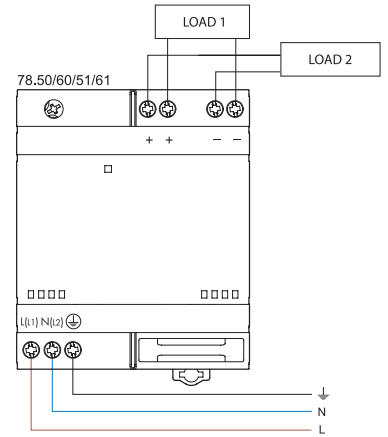
Conexiones básicas
